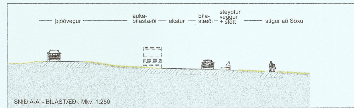
Skýringarmynd, bílastæði.
