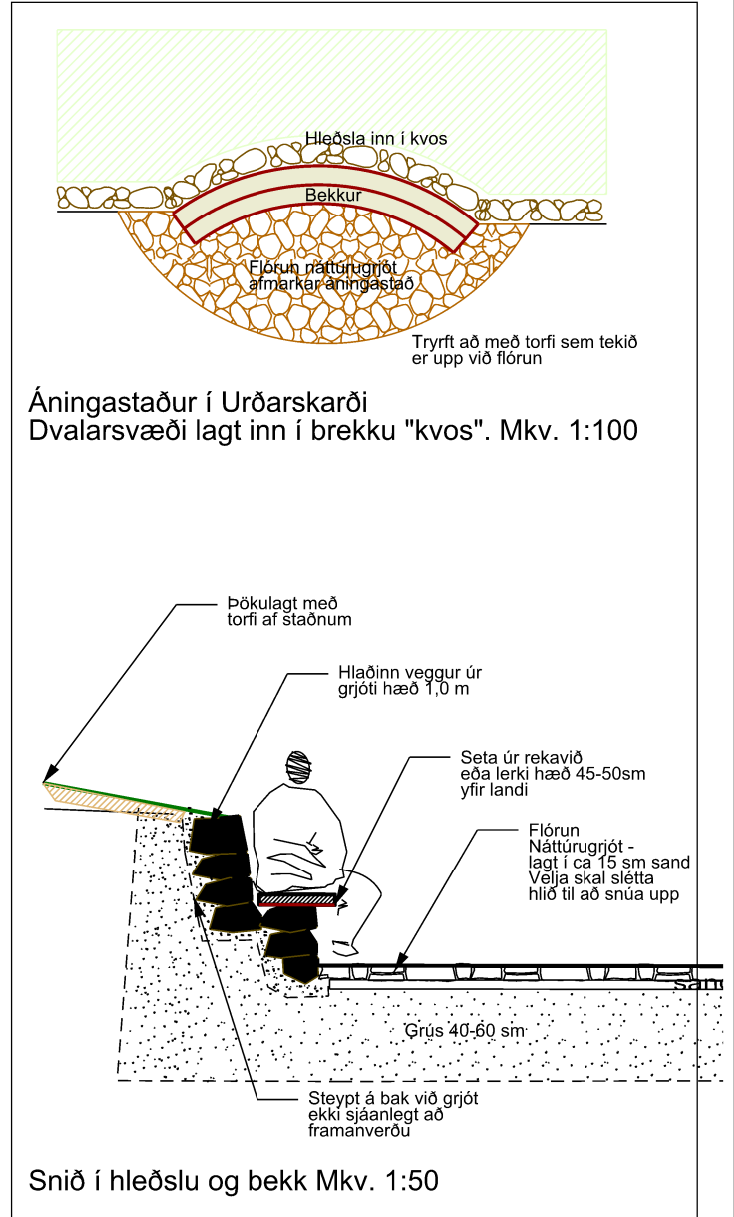
Áningastaður í Urðarskarði Grunnmynd og snið mkv. 1:100/1:50
