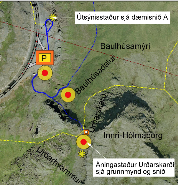
Þjónustuaðkoma og útsýnisstaður Afstöðumynd
